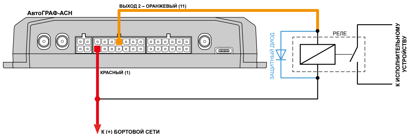
Рис.16. Подключение выхода.
