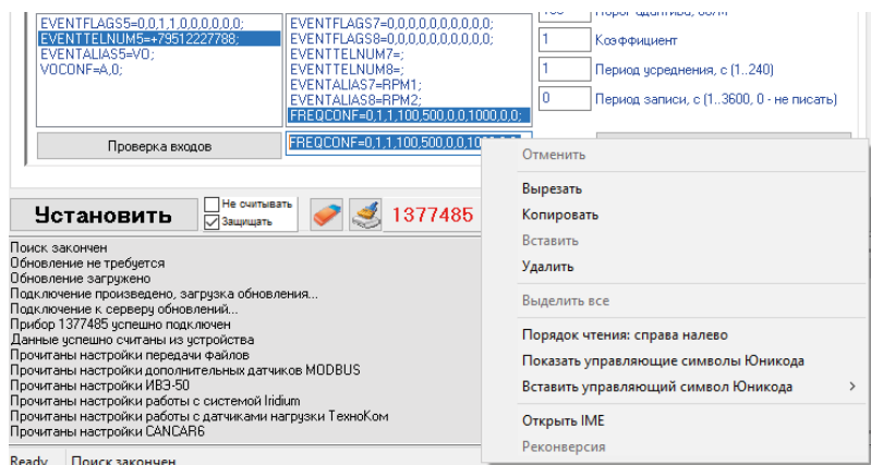
Рис.37. Копирование команды.
