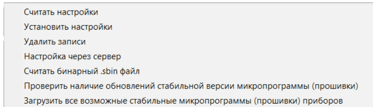
Рис.8. Меню «Устройство».
