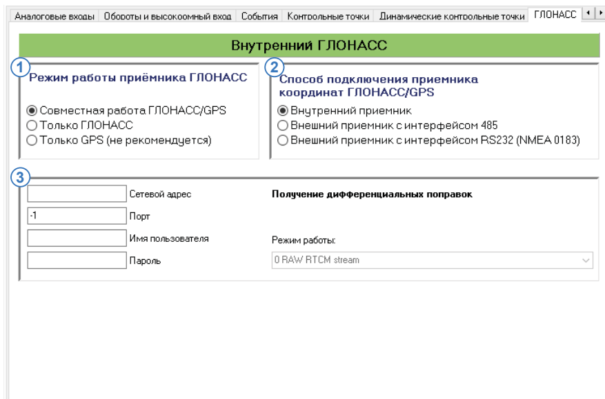
Рис.41. Вкладка «ГЛОНАСС».
