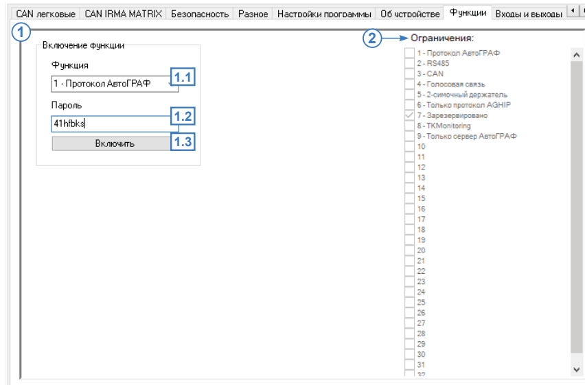
Рис.80. Вкладка «Функции».
