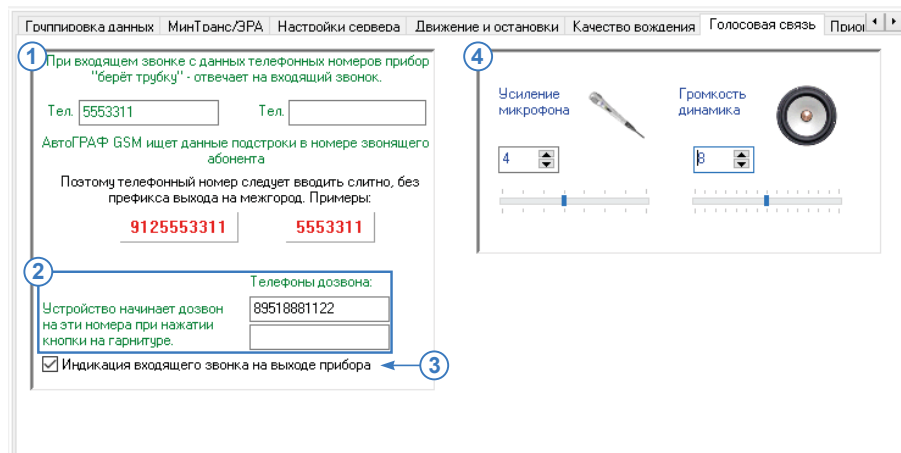
Рис.31. Голосовая связь.
