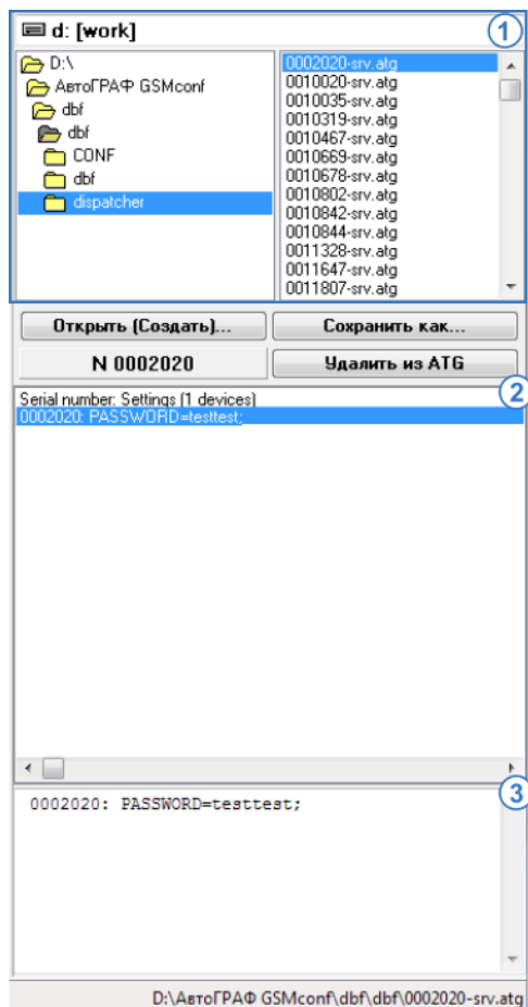
Рис.13. ATG браузер.
