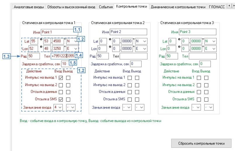
Рис.39. Контрольные точки.
